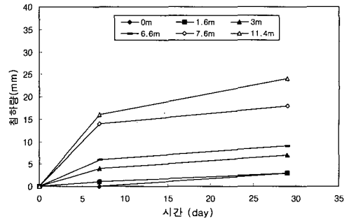
(a) 직선부
