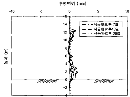
Fig. 5 벽체높이에 따른 보강토체내의 수평변위의 변화 (직선부)
