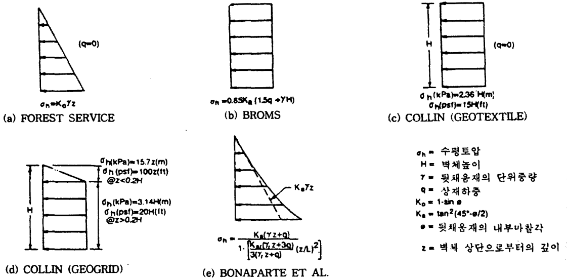
Fig. 1 타이백 방법에 사용된 토압분포
