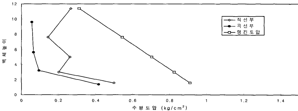
Fig. 3 벽체높이에 따른 블록배면의 수평토압의 변화 (시공완료 후 29일 경과시)
