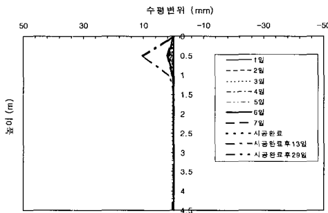
(b) 곡선부
