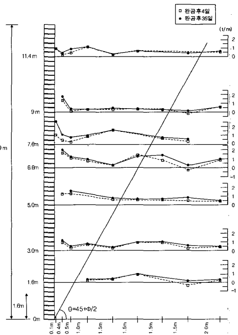
Fig. 9 벽체높이별 보강재의 유발인장력 변화
