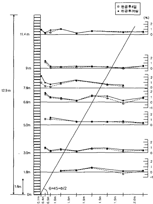
Fig. 8 벽체높이별 보강재의 유발변위 변화
