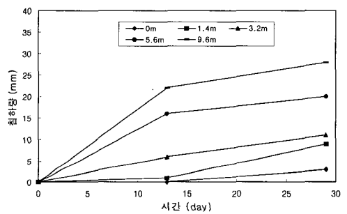
(b) 곡선부
