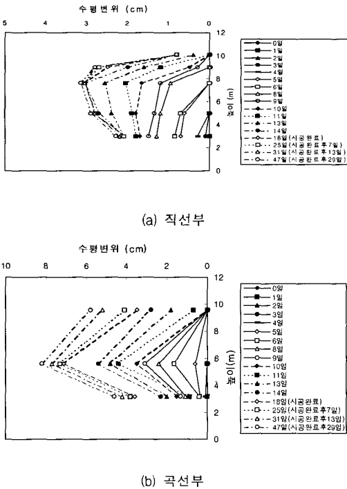
Fig. 4 벽체높이에 따른 블록배면의 수평변위의 변화
