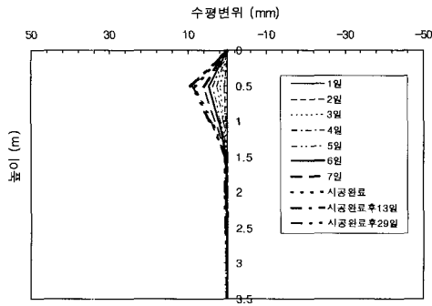
(a) 직선부
